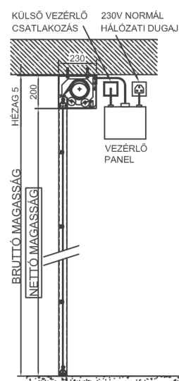
METSZETI RAJZ FALNYÍLÁSBA SZERELVE
