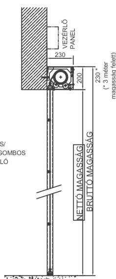
METSZETI RAJZ FALNYÍLÁS ELÉ SZERELVE
