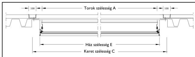
KERESZTMETSZET — FR KERETTÍPUSAL
